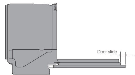
Installazione con porta sliding XL/XXL
