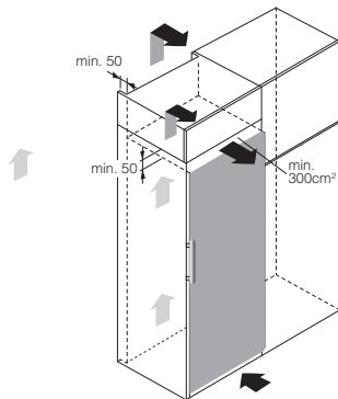
Ventilazione dell'apparecchiatura
