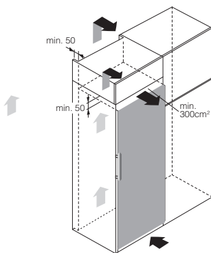
Ventilazione dell'apparecchiatura
