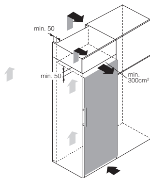
Ventilazione dell'apparecchiatura
